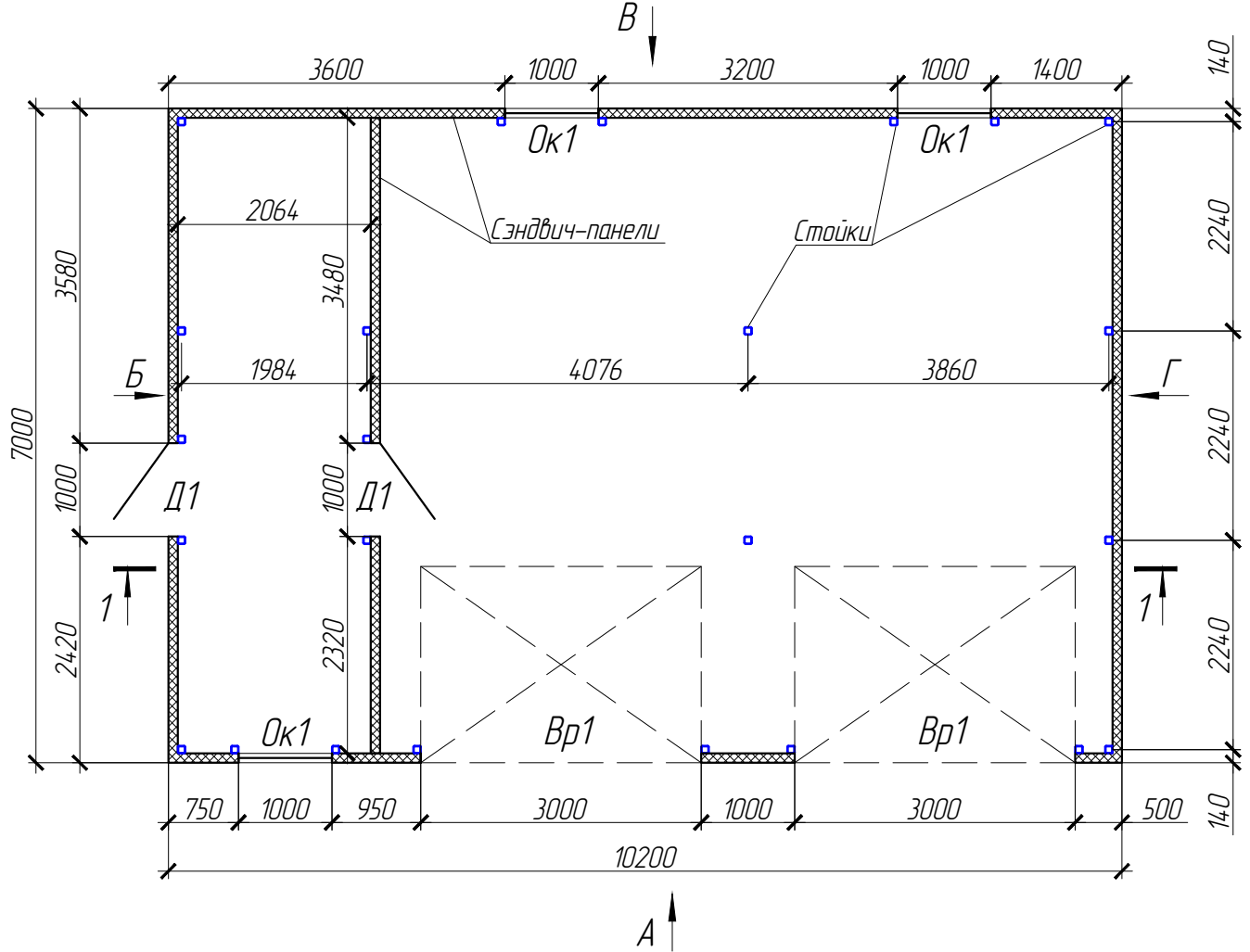
План гаража
